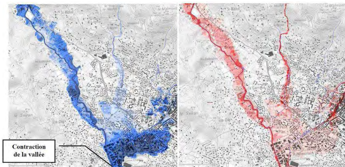
Figure 24 : Hauteur d'eau et vitesses d'écoulement –La Nartuby en amont de Salamandrier
